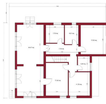
PIANO PRIMO
