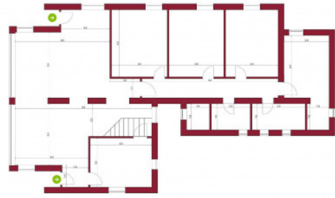
PIANO TERRA LE MISURE VANNO VERIFICATE IN SEDE DI RILIEVO
