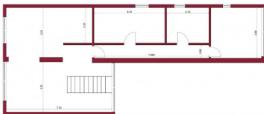
PIANO PRIMO LE MISURE VANNO VERIFICATE IN SEDE DI RILIEVO
